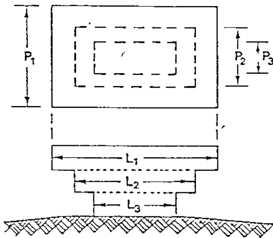
Aire de bâtiment L_1 \times P_1
