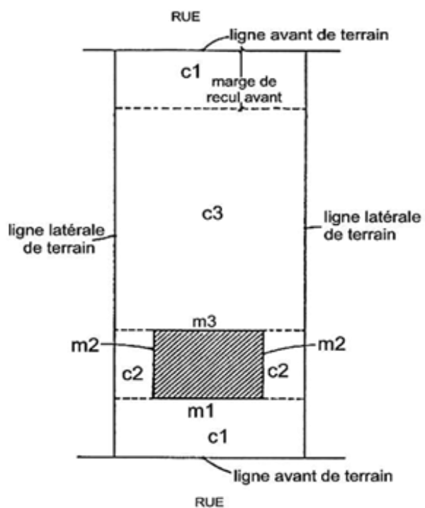
terrain intérieur transversal
